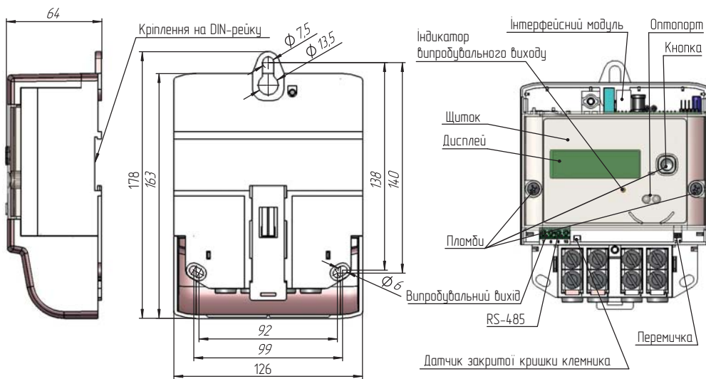
Малюнок А.1 - Загальний вигляд, габаритні і установчі розміри, місця установки пломб на корпусі однофазного лічильника типу MTX 1A10.D...2...0-...4
